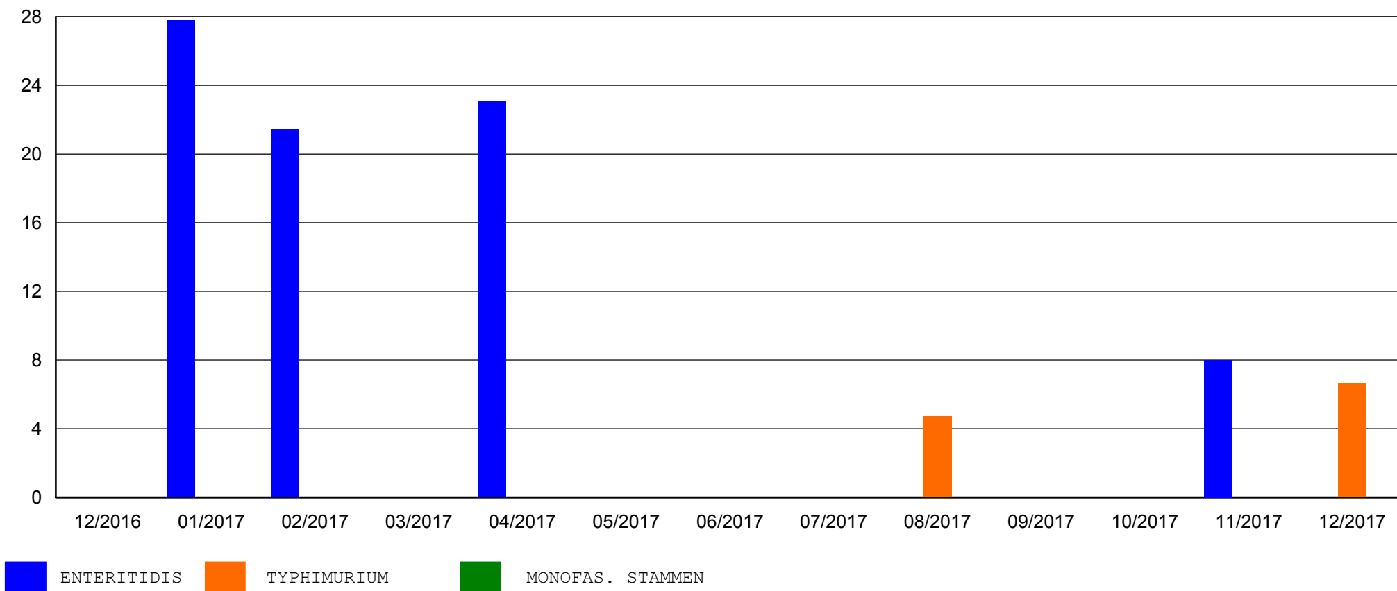
% Pos ENTERIDIS & TYPHIMURIUM & MONOFAS. STAMMEN
